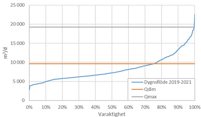
Figur 3 Histogram över avloppsvattenflödet till Överstatorp ARV (2019-2021).
