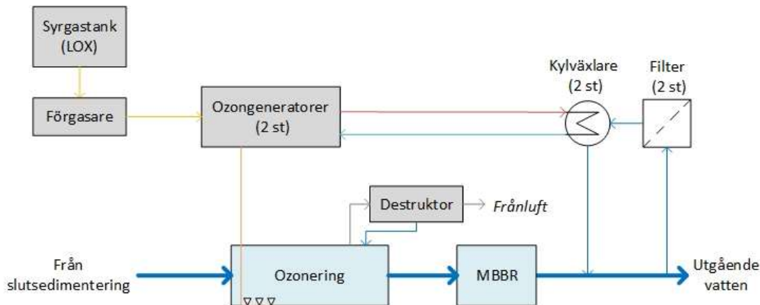
Figur 7 Blockschema över föreslagen ozoneringsprocess för rening av mikroföroreningar vid Överstatorp ARV.
