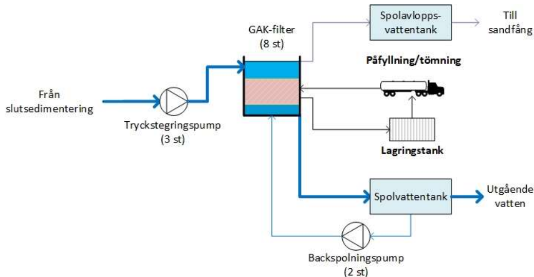
Figur 9 Blockschema över föreslagen GAK-anläggning för rening av läkemedel och andra mikroföroreningar vid Överstatorp ARV.
